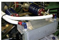
オイルクーラー配管
