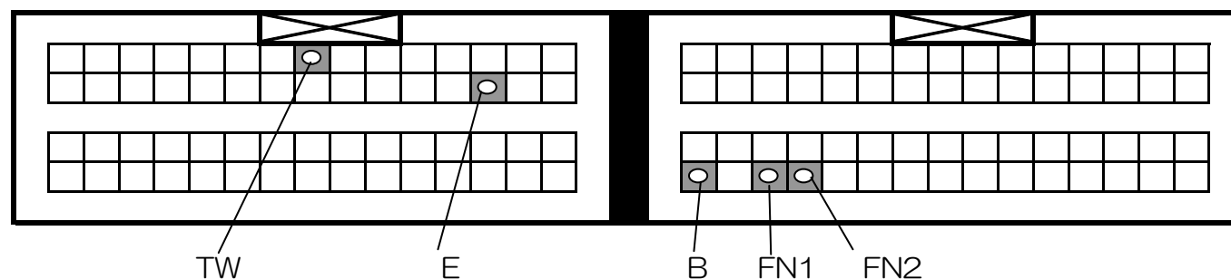
MAZDA デミオ DE#FS ECU配列図
